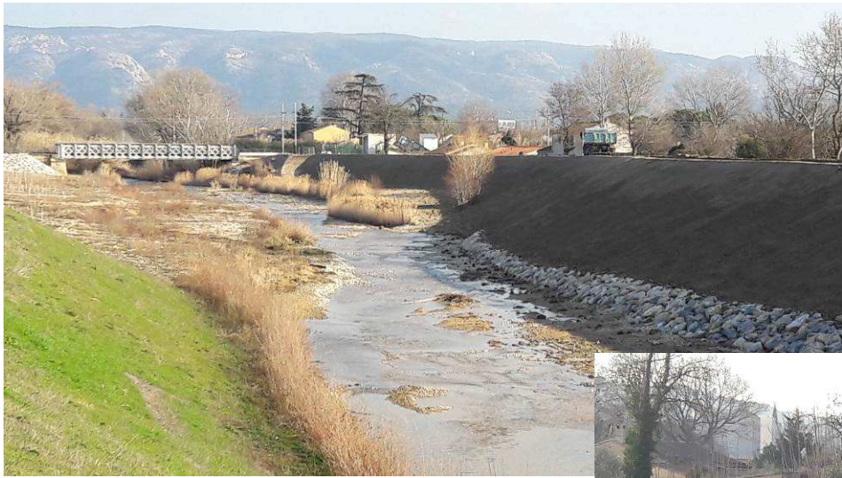
Nappage des talus de terre végétale et retalutage
